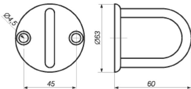
защелка настенная для каната SW 060.102
