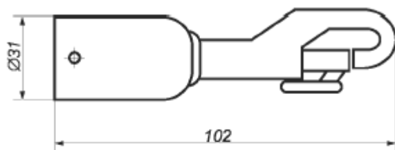
защелка настенная для каната SW 060.102
